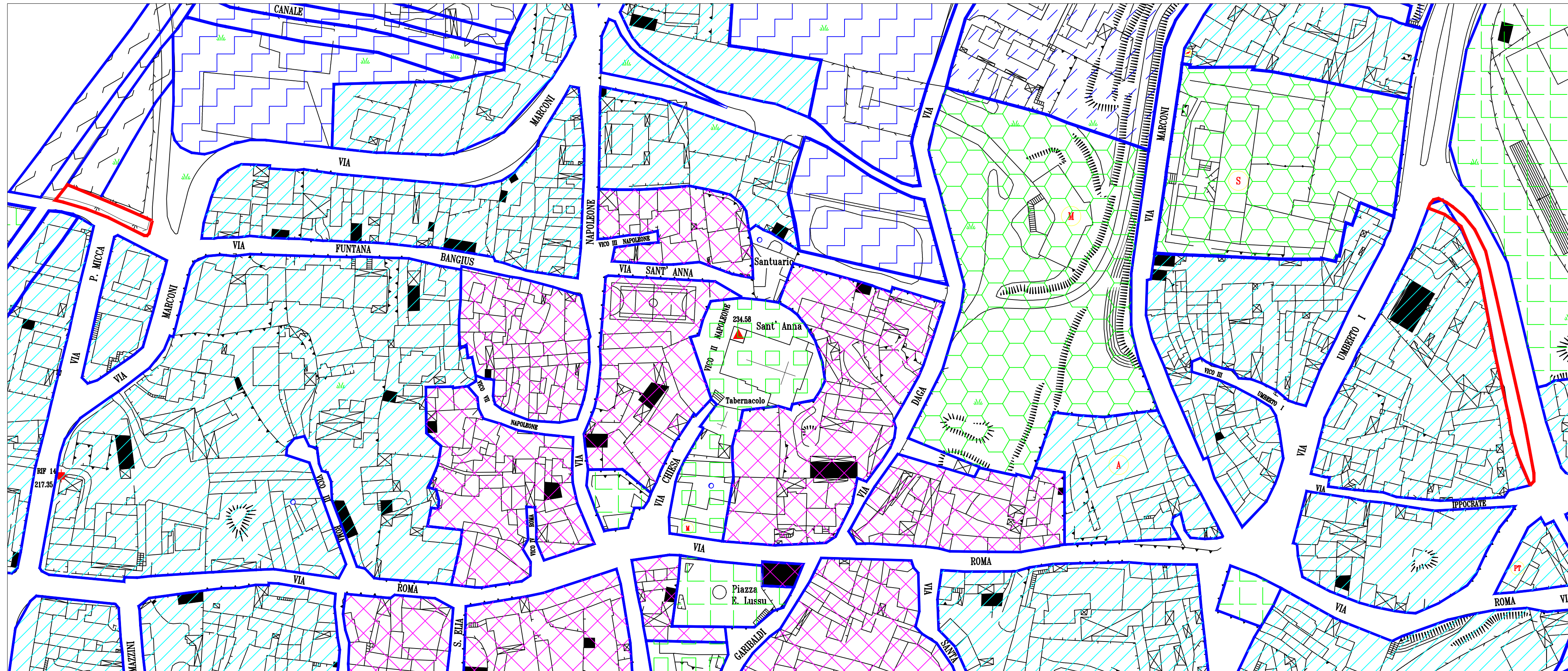
Stralcio PUC del Comune di Selegas - 1:1000
